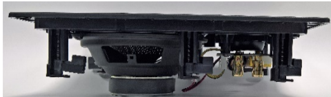
Seulement 3 1/8 "de profondeur pour s'intégrer facilement dans n'importe quel mur.
